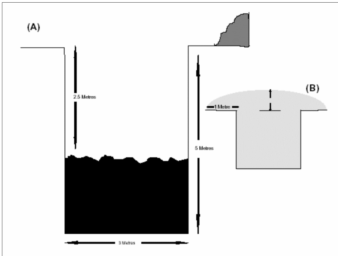
Poprečni presjek jame za zbrinjavanje leševa uginulih životinja i drugog životinjskog otpada (ABP) zakopavanjem
