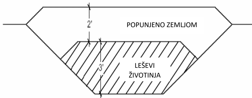
Poprečni presjek rova za zbrinjavanje leševa uginulih životinja i životinjskog otpada (ABP) zakopavanjem
