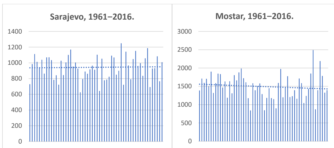
Slika 8: Trendovi promjena padavina u Federaciji BiH, 1961–2016. (Sarajevo, Mostar)
