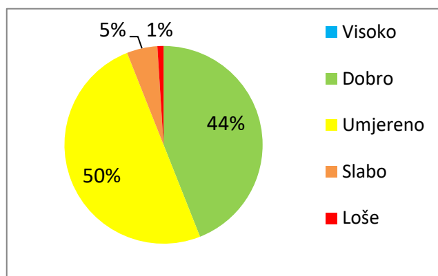
Slika 1: Ekološko stanje VT-a površinskih voda, po monitoringu na vodnom području rijeke Save) (Agencija za vodno područje rijeke Save 2021)
