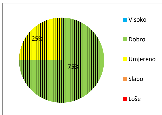
Slika 5: Ekološki potencijal jako izmijenjenih i umjetnih vodnih tijela površinskih po monitoringu na vodnom području Jadranskog mora (2016-2019)
