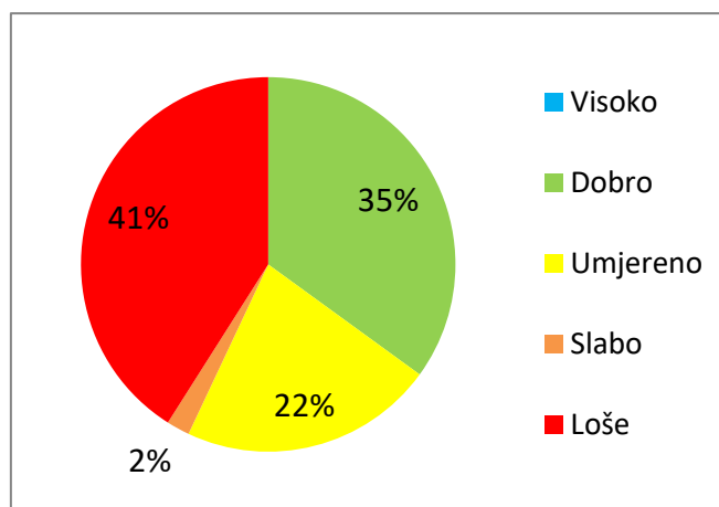
Slika 3: Ukupna ocjena stanja vodnih tijela površinskih voda, po monitoringu na vodnom području rijeke Save (2011-2018)
