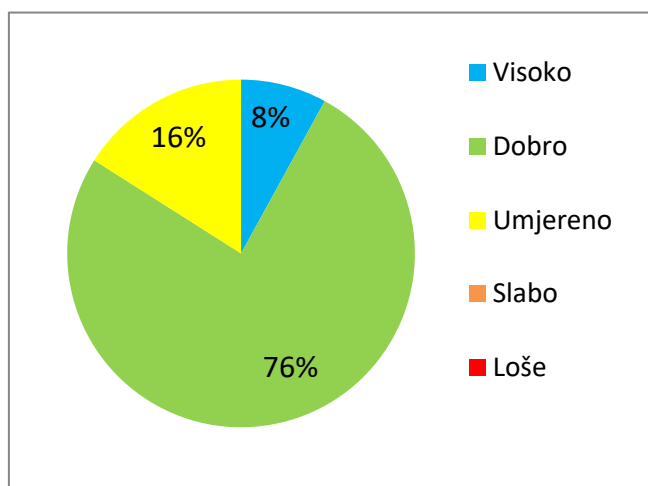
Slika 4: Ekološko stanje prirodnih vodnih tijela površinskih voda po monitoringu na vodnom području Jadranskog mora (2016-2019) (Agencija za vodno područje Jadranskog mora 2021)
