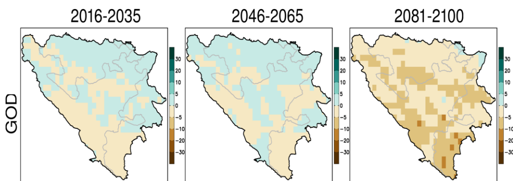
Slika 10: Očekivane promjene padavina u BiH prema scenariju RCP8.5
