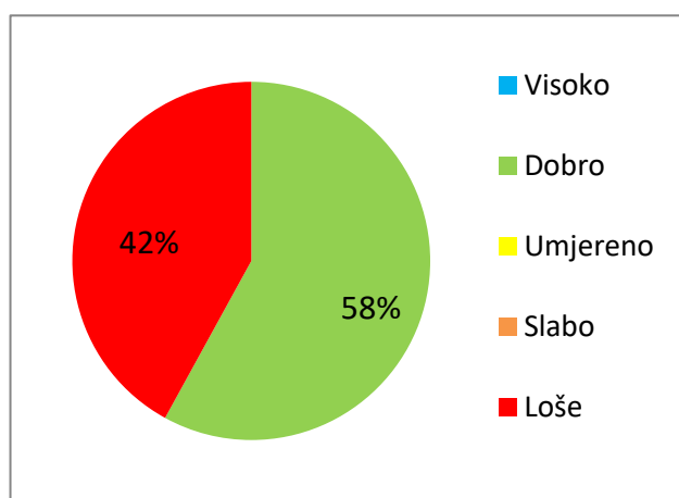
Slika 2: Hemijsko stanje vodnih tijela površinskih voda, po monitoringu na vodnom području rijeke Save (2011-2018)
