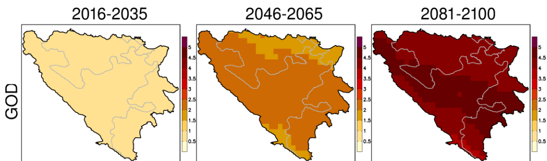
Slika 9: Očekivane promjene temperature zraka u BiH prema scenariju RCP8.5
