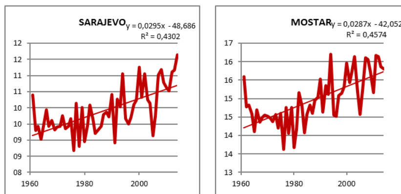
Slika 7: Trendovi promjena temperature zraka u Federaciji BiH, 1961–2016. (Sarajevo, Mostar)
